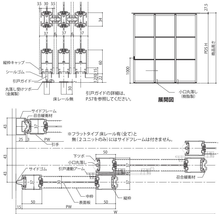
横断面図
