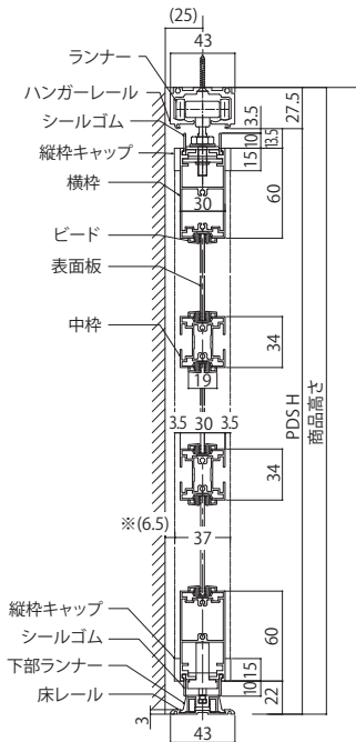
縦断面図
