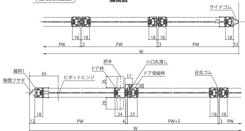
横断面図
