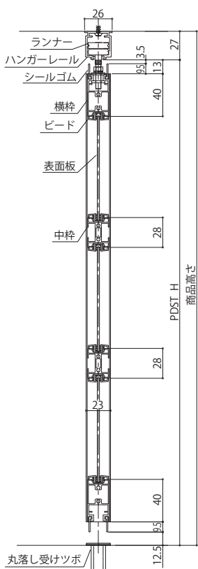
縦断面図
