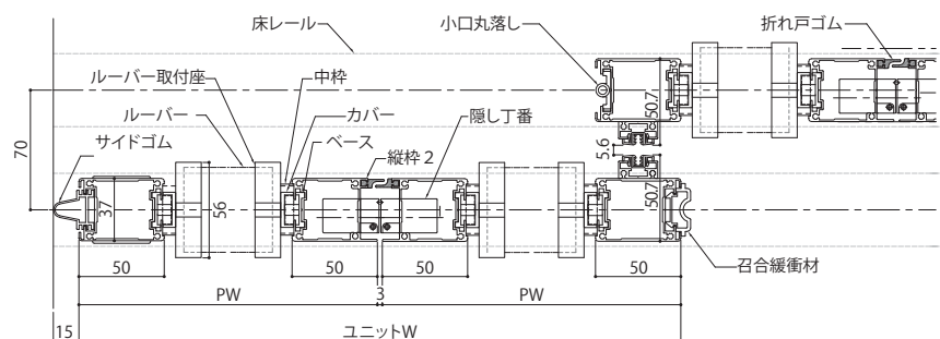
横断面図
