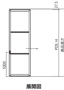
展開図
