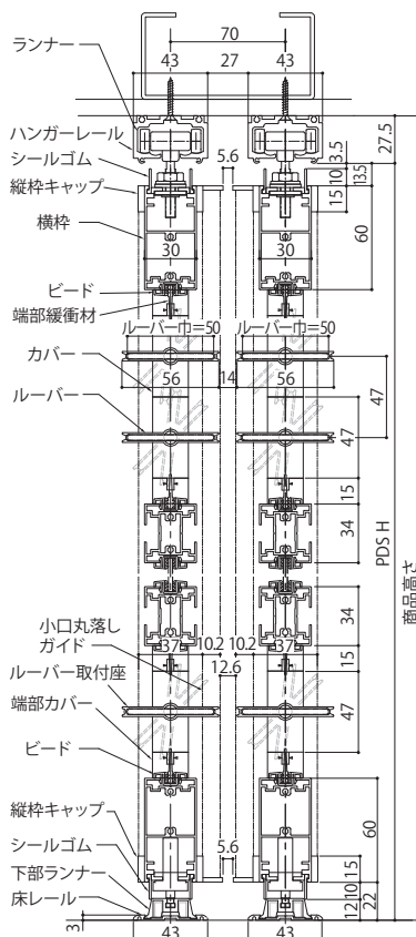
縦断面図
