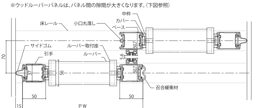
横断面図
