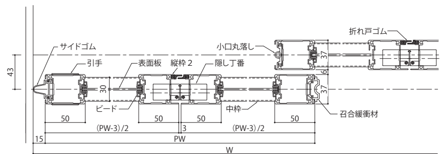
横断面図
