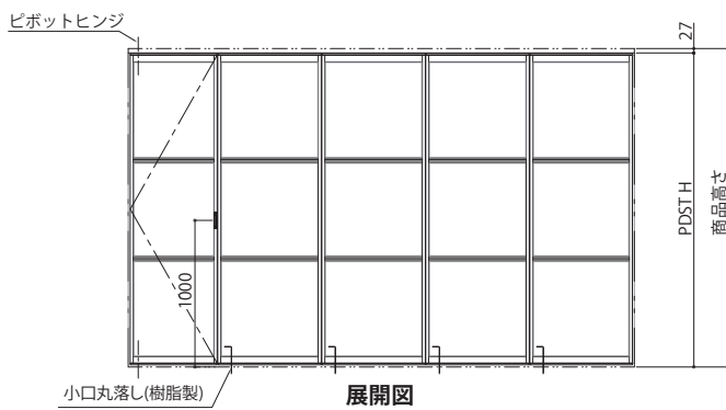
展開図
