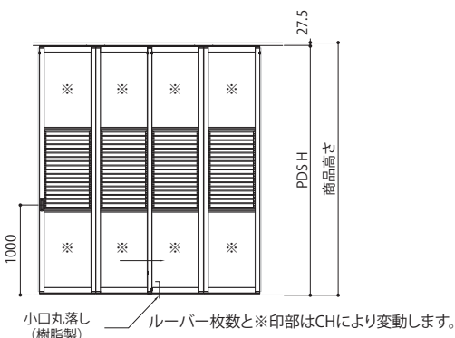
展開図
