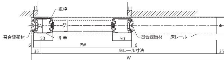
横断面図
