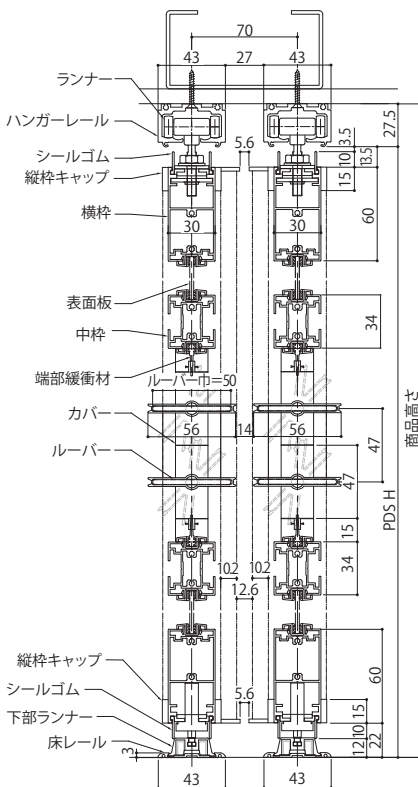
縦断面図
