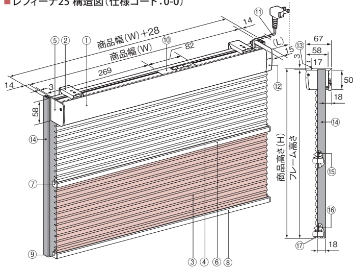
■レフィーナ25 構造図(仕様コード:0-0)
