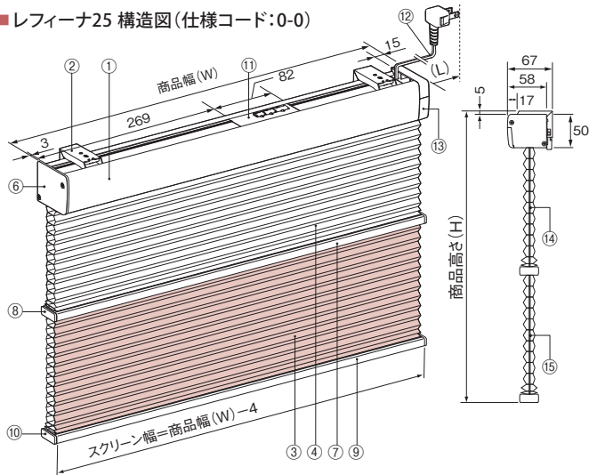
■レフィーナ25 構造図(仕様コード:0-0)
