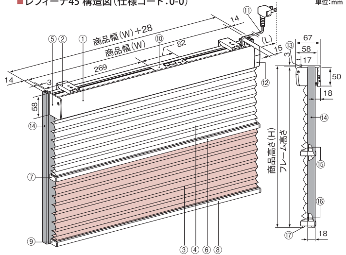
■レフィーナ45 構造図(仕様コード:0-0)
