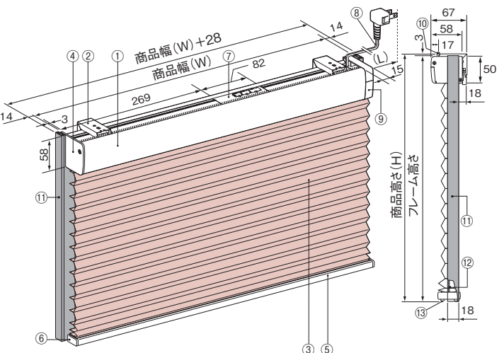
■レフィーナ45 構造図
