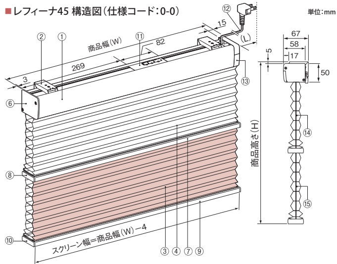
■レフィーナ45 構造図(仕様コード:0-0)
