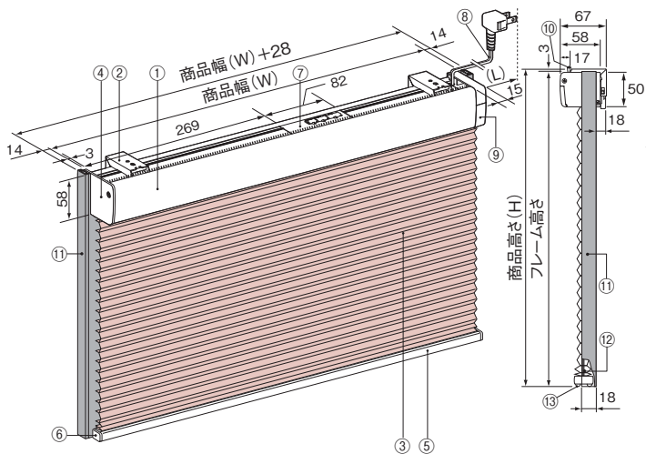
■レフィーナ25 構造図
